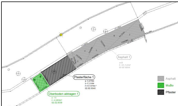
Ausdruck Aufmaßzeichnung
