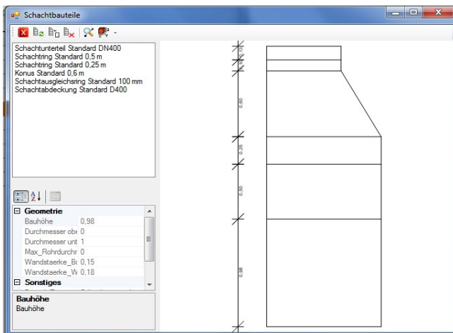
Bild: Automatische Erzeugung der Schachtbauteile.
